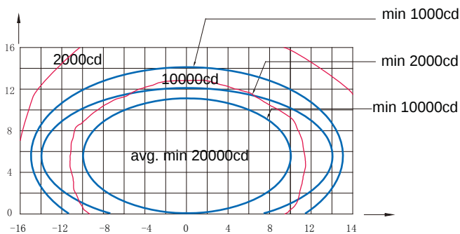
进近中线灯(白光)，ICA0图A2-1 (主光束垂直覆盖范围0°—11°)
