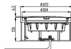
图2. 12吋浅桶底座安装
