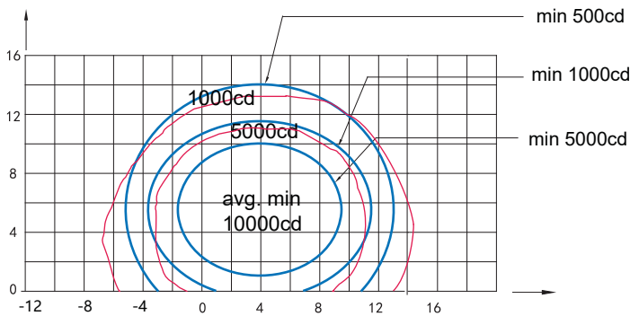
跑道入口/末端灯(绿光), ICAO 图A2-3
