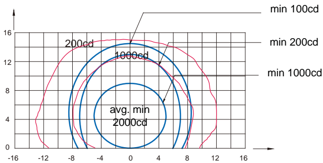
快速出口滑行道指示灯(黄光), ICAO 图A2-7
