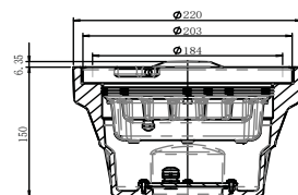
图1. 8吋浅桶底座安装
