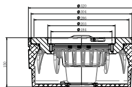
图2. 利用12吋/8吋过渡圈安装在12吋浅桶底座上
