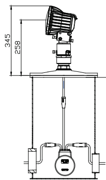
图1. 12吋深桶底座安装
