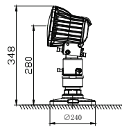
图2. 法兰盘直接安装
