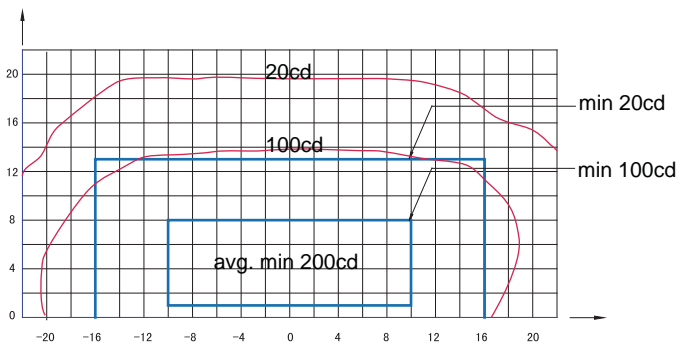
中间等待位置灯(黄光), ICAO图A2-12
