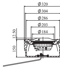
图2. 利用12吋/8吋过渡圈安装在12吋浅桶底座上
