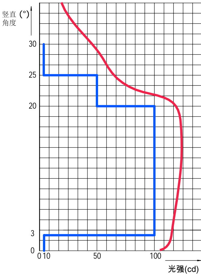
LED瞄准点灯(白光), AC-137-CA 5.2.1.6章节 (主光束垂直覆盖范围0°—30°)
