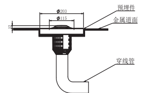
预埋管安装
