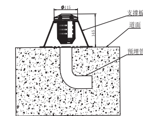
混凝土道面嵌入式安装
